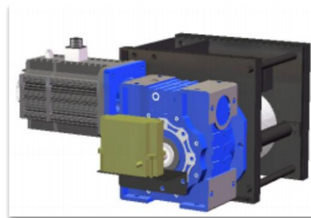
一体式双吊点自动排绳升降机
